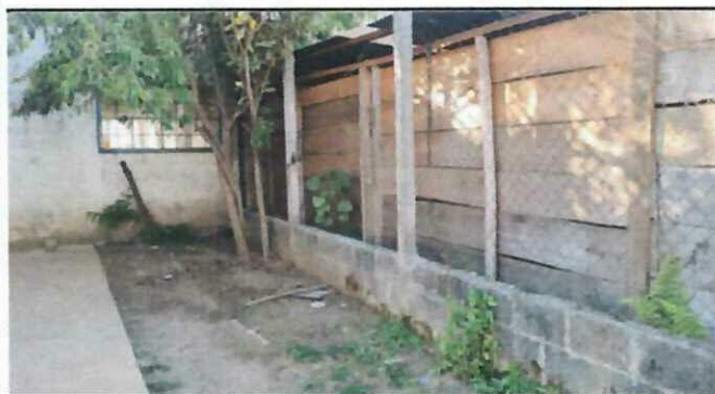
Foto 3: Construcción de 25 mts. lineales por 3.70 mts. de altura que equivale a 92.50 mts.2 de muro perimetral en la parte lateral de la escuela
