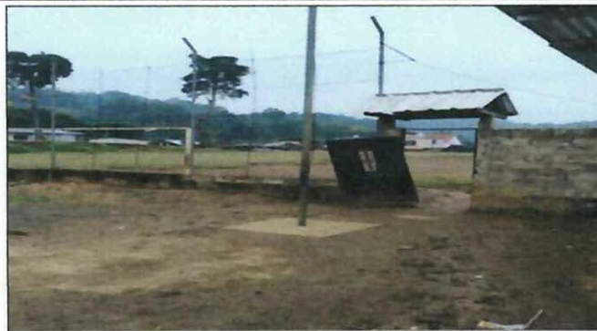
Foto 2: Construcción de 33 mts. lineales por 3.70 mts. de altura que equivale a 122.10 mts.2 de muro perimetral en la parte de atrás de la escuela
